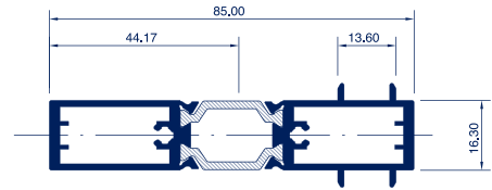
Ref. 4337 · Unión
