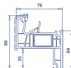
Ref. 101.358 Refuerzo 113.019 Marco con solapa SL76
