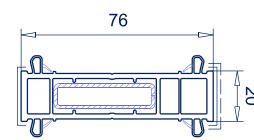
Ref. 116.230 Unión de marcos SL76, 26 mm
