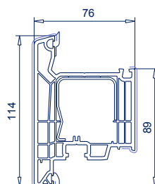
Ref. 103.386 Refuerzos 113.270, 113.368 & 115.003. Apertura hacia afuera Hoja SL76
