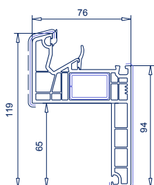
Ref. 101.359 Refuerzo 113.019 Marco renovación
