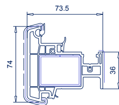
Ref. 102.356 Refuerzo 113.001 Batiente SL 76
