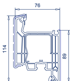
Ref. 103.385 Refuerzos 113.270, 113.368 & 115.003 Hoja SL76
